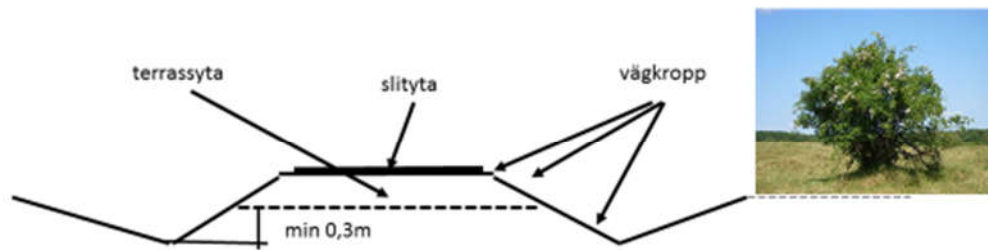
Tvärsektion av väg med godtagbart dikesdjup
